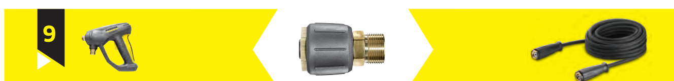
EASY!Lock orientabile - M 22x1,5 Codice 4.111-046.0 Adattatore girevole per collegare tubi alta pressione con filetto M 22x1,5 con pistole alta pressione EASY!Force
